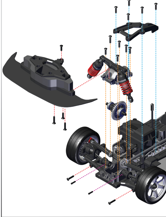
Ausbau des vorderen Differentials
