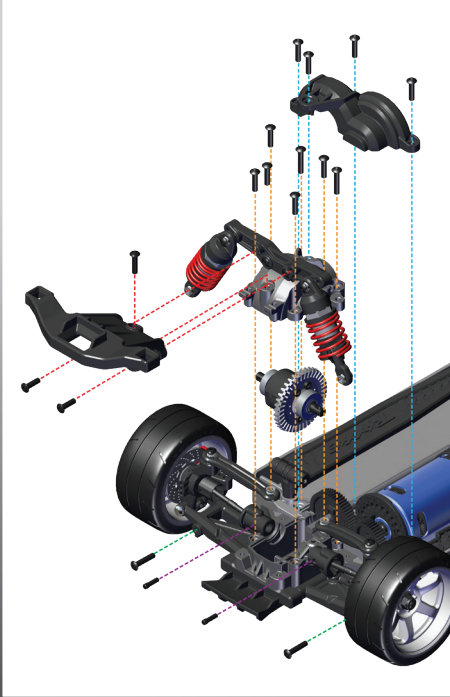
Ausbau des hinteren Differentials
