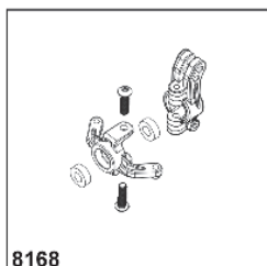
8168 Radträger links
