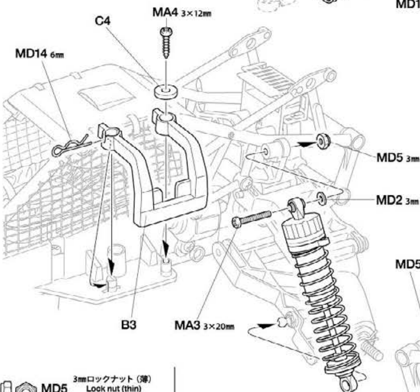
MD2 3mm ワッシャー Washer Beilagscheibe Rondelle
