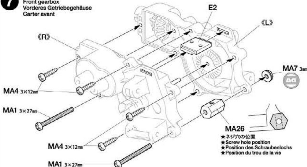
MA4 3x12mmタッピングビス Tapping screw Schneidschraube Vis taraudeuse
