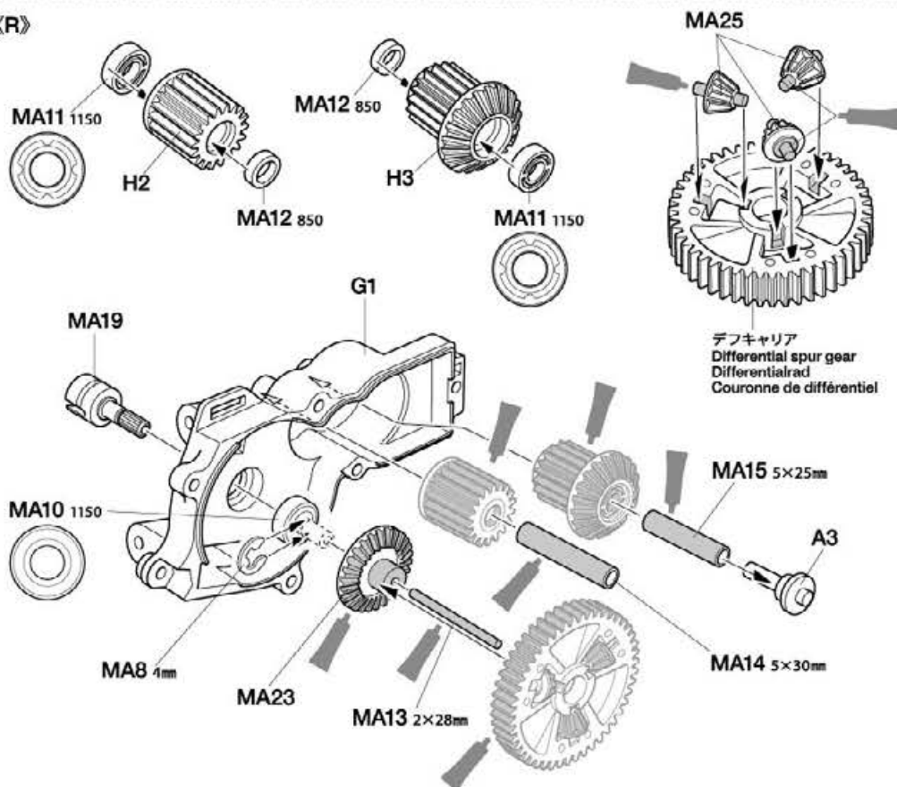
MA25 ベベルギヤ S Small bevel gear Kegelrad klein Petit pignon conique
