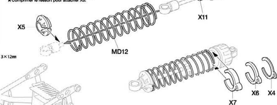
MA4 3×12mm タッピングビス Tapping screw Schneidschraube Vis taraudeuse
