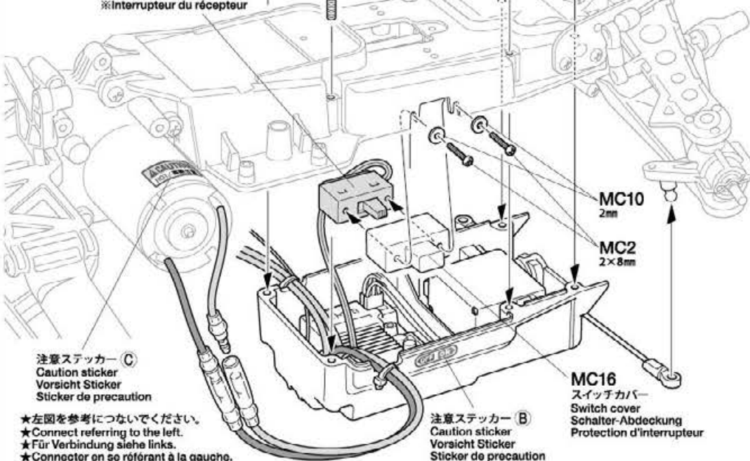
MC2 x2 2x8mm丸ビス Screw Schraube Vis
