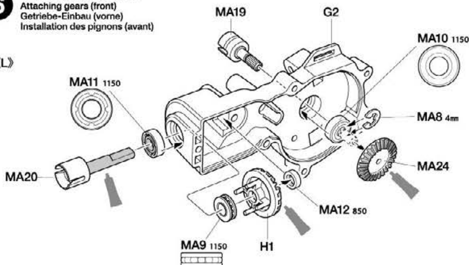
MA9 1150スラストベアリング Ball thrust bearing Druckkugellager Butée à billes
