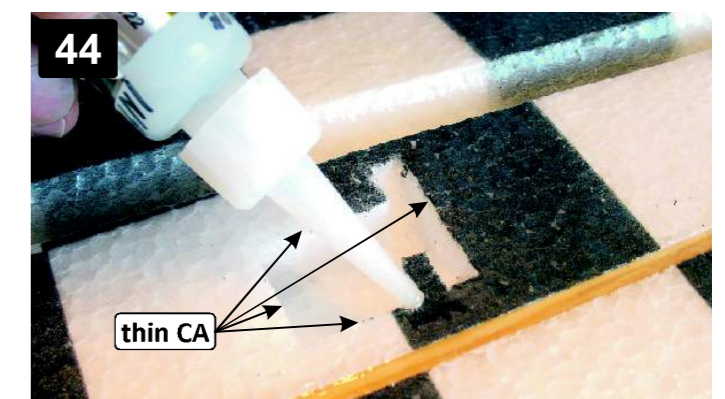
44 Hrany fólie přilepte k polovinám křídél (2, 3) řídkým CA lepidlem. Glue edges of cropped covering foil to the wing (2, 3) with thin CA.
