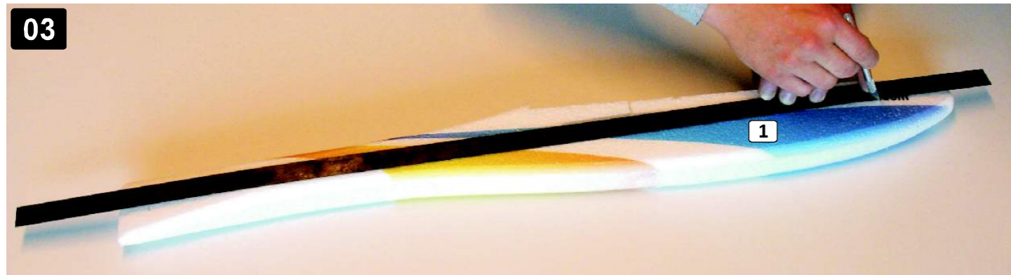
03 Podél pravítka prořízněte drážku pro výztuž (26). Hloubka 3mm. Řez provedte z obou stran trupu. Cut the slot along a ruler. Slot must be 3mm deep. Cut both sides of fuselage.
