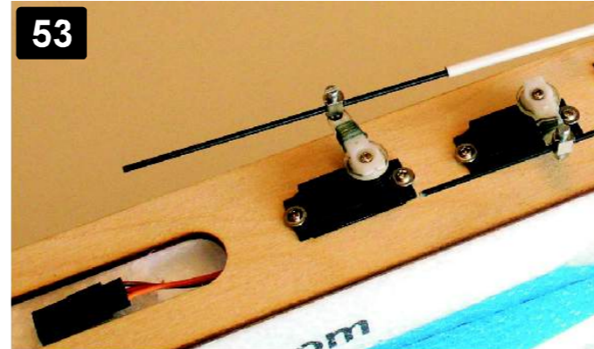
Nainstalujte serva ocasních ploch. Vložte je do otvorů v desce kabiny (8) a kabelky protáhněte do prostoru pro přijímač v zadní části kabiny. Serva přišroubujte. Put rudder's and elevator's servos to the wooden former (8).
