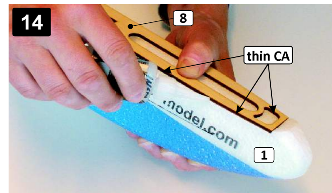
14 Na lanovody (30, 31) nasadte desku kabiny (8), přitlačte ji k přední hraně trupu a přilepte ji řídkým CA lepidlem k přední části trupu (1). Použijte aktivátor lepidla. Put the former (8) on the tubes (30, 31). Push former (8) to the forepart of fuselage (1) and glue it in front with thin CA. Use activator spray.
