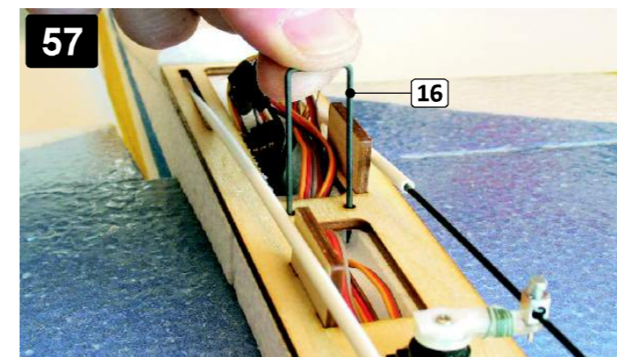
Zajistěte poloviny křídla (2, 3) proti vysunutí kovovou sponou (16). Sponu vložte do otvorů v desce kabiny (8). Fix wing panels together with former (16). Put it to the holes in the woden plate (8).
