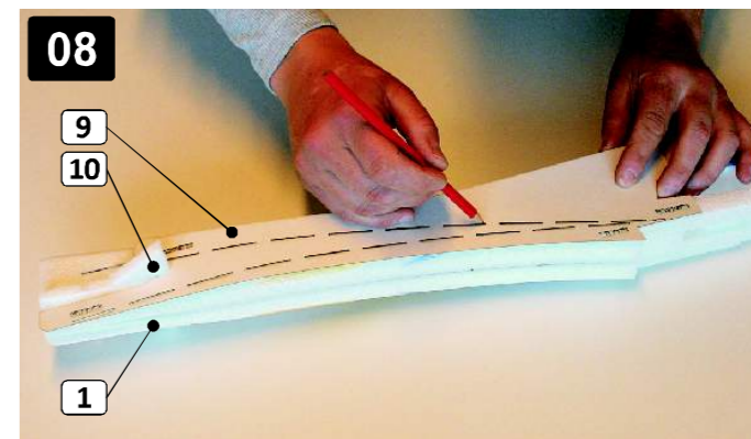
08 Do trupu (1) vložte střední díl VOP (10) a na levou stranu trupu přiložte šablonu (9). Tužkou vyznačte vedení lanovodu VOP (31). Insert middle part of elevator (10) to the fuselage (1). Attach the template (9) to the left side of fuselage. Use pencil to draw position of plastic tube (31).
