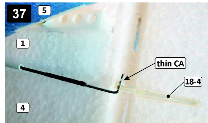
37 Táhlo SOP (28) připojte na páku SOP (18-4) a zajistěte jej plastovou podložkou (18-7). Podložku přilepte kapkou řídkého CA lepidla k drátěné koncovce (21). Connect rudder push rod (28) to the rudder horn (18-4). Put on the plastic former (18-7) into the "L" wire (21) and fix it with small drop of thin CA.
