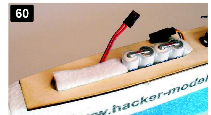
Po vyvážení modelu vydlabejte v trupu lože pro přijímačové baterie. Baterie v otvoru zajistěte např. kouskem polystyrenu nebo molitanu. After finding right position of CG cut off foam from the front part of fuselage to place accu. Fix accu in position with polystyrene etc.
