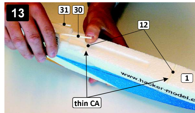
13 Do drážek v trupu (1) vlepte řídkým CA lepidlem trubičky pro čepy kabiny (12). Použijte aktivátor ve spreji. With thin CA glue the tubes (12) to the grooves at the fuselage (1). Use activator spray.
