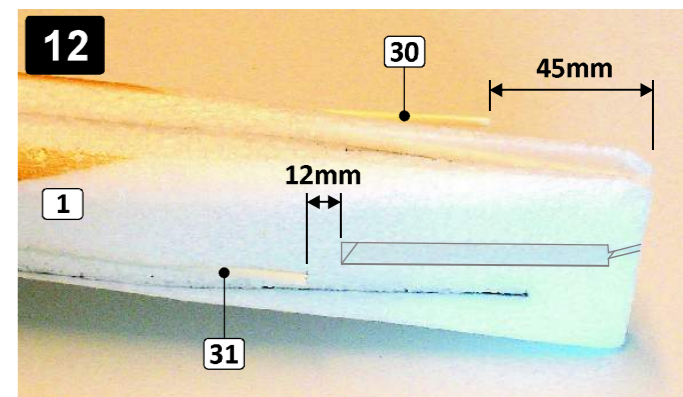
12 Zatlačte lanovody SOP a VOP (30, 31) do drážek. Zatím nelepte! Zalepíte je až po úplném dokončení modelu a nastavení vychylek kormidel. Push the tubes (30, 31) to the fuselage (1). Don't glue them now! You will glue them after completion the plane and all settings.
