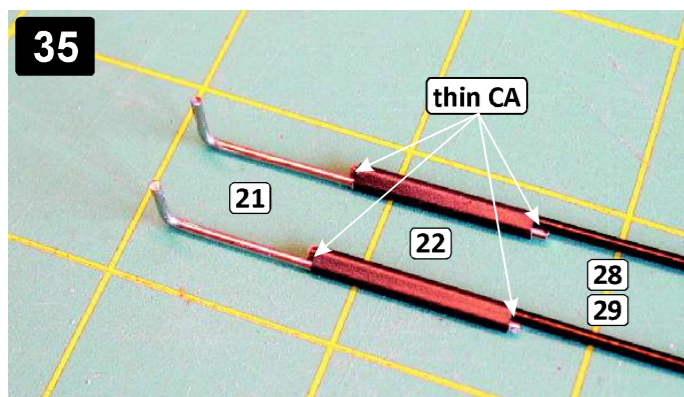
35 Táhla ocasních ploch (28, 29) jsou na jedné straně zakončena koncovkou "L" (21). Na táhlo nasadte smršťovací bužírku (22), do bužírky vložte drátěnou koncovku "L" (21) a ohřátím bužírku stáhněte (zapalovačem nebo horkovzdušnou pistolí). Konce bužírky zajistěte zakápnutím řídkým CA lepidlem. Elevator and rudder push rods have "L" ending (21) at one of his side. Insert push rod (14, 15) and "L" wire (21) into the heat shrink tube (22) and heat up the tube (use lighter or heating gun). Fix rods using thin CA glue.
