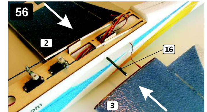
Poloviny křídla (2, 3) nasadte na spojku (16) a zasuňte je až k žebru (14) vtrupu. Attach the wing panels (2, 3) to the wire (16). Press them to fit central rib (14).
