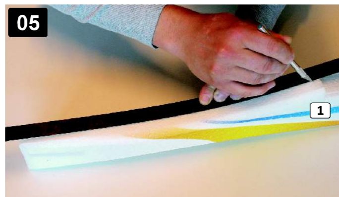
05 Prořízněte drážku pro výztuž (27). Hloubka 3mm. Cut the slot. The slot must be 3mm deep.
