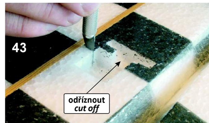
43 V polovinách křídél (2, 3) upravte otvory pro serva. Prořízněte zárez pro patky. Adjust openings for servos in the wing (2, 3).
