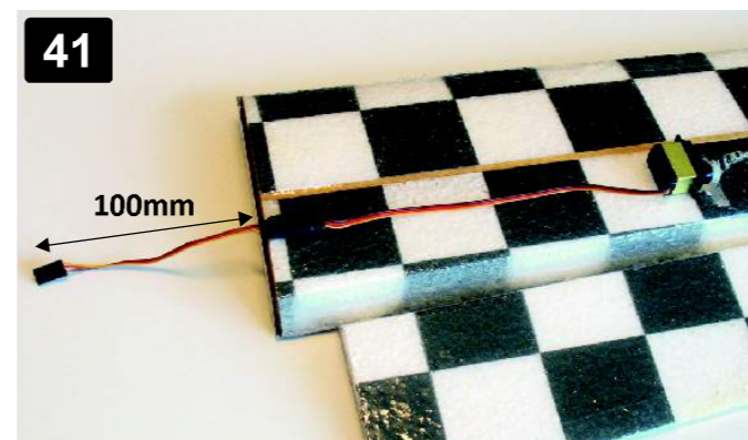
41 Zkontrolujte délku kabelu serv křídélek a případně jej prodlužte. Spoj zajistěte např. smršťovací bužirkou proti rozpojení. Check length of servo cable, use extension to have right length. Fix connection with shrink tube or self-adhesive tape.
