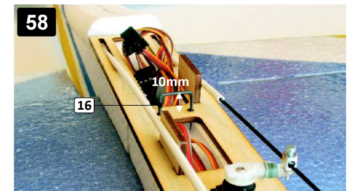
Sponu (16) zatlačte do trupu (1). Spona propíchně křídlo. Při rozebírání modelu nezapomeňte sponu vyjmout! Press former (16) to the fuselage (1). Former will pierce the wing. Don't forget to remove former (16) before removing wing panels!
