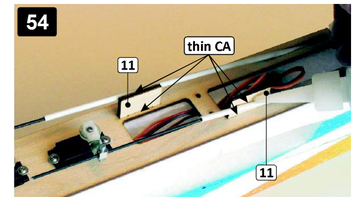
Do desky kabiny (8) zalepte řídkým CA lepidlem držáky lanovodů (11). Lanovody (30, 31) přilepte k držákům (11). Glue wooden formers (11) with the plate (8) with thin CA. Glue the rudder's and elevator's guide rods to the wooden formes (11).
