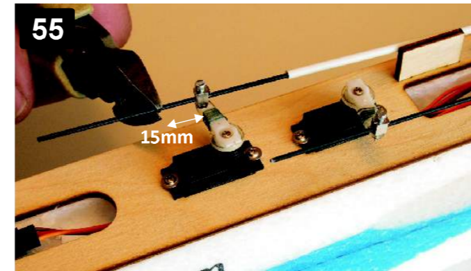
Zkraťte táhla s přídatkem cca 15mm. Cut elevator's and rudder's push rods now! Keep 15mm overlap.
