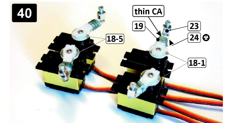
40 Plastové páky prodloužení (18-1, 18-5) přilepte kapkou řídkého CA lepidla k páce serva. Spoj omotejte 5-6 závitů nitě (19), zalepte CA lepidlem a přesahující nit odřízněte. Nasaďte konektory táhel (23) a zajistěte je podložkami quicklock (24). Páky nasadte na serva.
