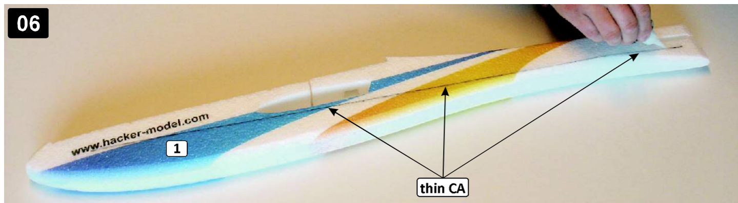
06 Výztuhu (26) zalepte řídkým CA lepidlem do trupu (1). Výztuhu zalepte z obou stran trupu. Po cca 5ti minutách přestříknete lepený spoj aktivátorem. Glue up the glass (26) to the fuselage (1) with thin CA. Glue it on both sides of fuselage. Use activator spray after 5 minutes.
