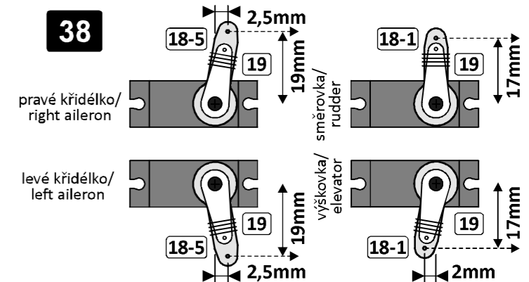
38 Schéma osazení pák na servech. Pro veliké výchylky na kormidlech (akrobatické nastavení) použijte prodloužení pák (18-1, 18-5). Scheme of servo arms. For large movements of the control surfaces (aerobatic settings) use the arm extensions (18-1, 18-5).
