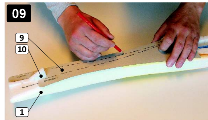
09 Na pravou stranu trupu přiložte šablonu (9). Tužkou vyznačte vedení lanovodu SOP (30). Vyjměte střední díl VOP (10) z trupu. Attach the template (9) to the right side of fuselage. Use a pencil to draw position of plastic tube (30). Take out former (10).
