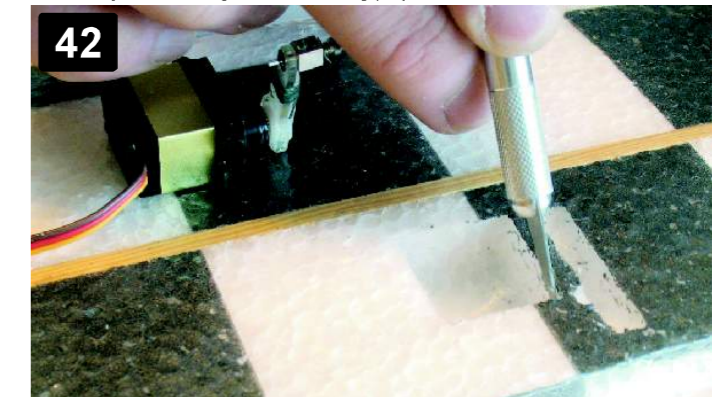
42 Odřízněte fólii nad otvory pro serva křídélek v polovinách křídla (2, 3). Cut off the foil around the edges of the holes for aileron servos.
