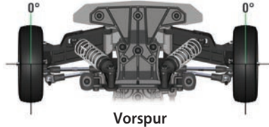
Vorspur
