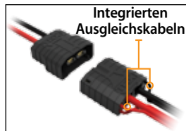
Traxxas Hochstromanschluss (4S) mit iD und integrierten Ausgleichskabeln
