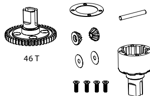
500405592 Centerdiff complete Mitteldiff komplett
