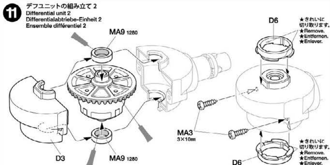
MA3 ×2 3×10mmタッピングビス Tapping screw Schneidschraube Vis taraudeuse
