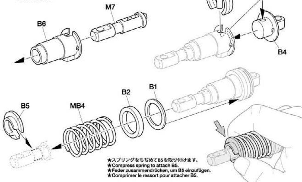
MB4 コイルスプリング ×4 Coil spring Spiralfeder Ressort hélicoïdal
