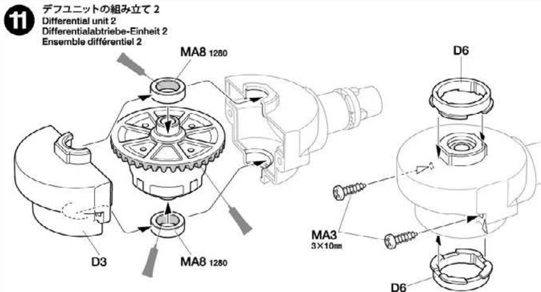
MA3 ×2 3×10mmタッピングビス Tapping screw Schneidschraube Vis taraudeuse
