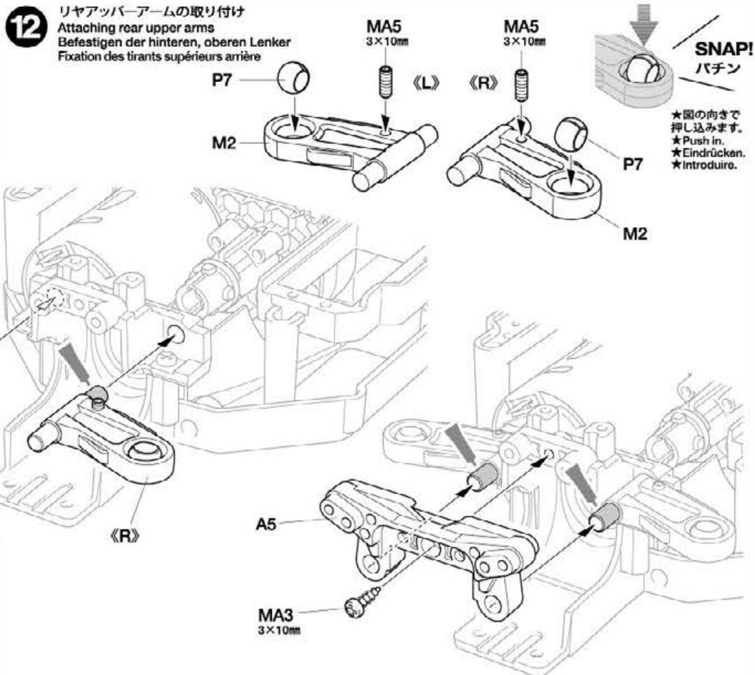
MA3 ×1 3×10mmタッピングビス Tapping screw Schneidschraube Vis taraudeuse
