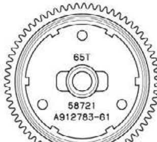
GB4 65T スパーギヤ 65T Spur gear 65Z Hauptzahnrad Couronne 65 dents
