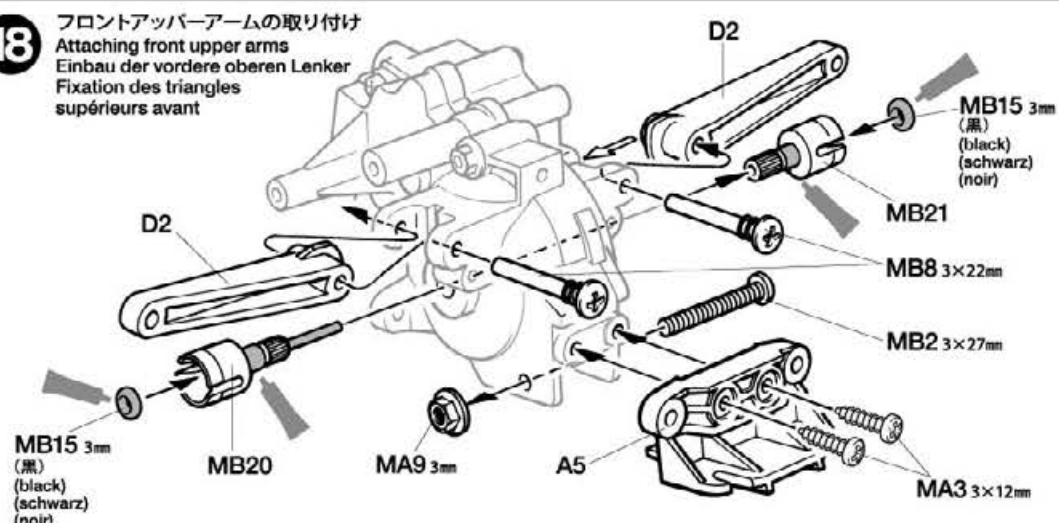
MA3 x2 3×12mm タッピングビス Tapping screw Schneidschraube Vis taraudeuse
