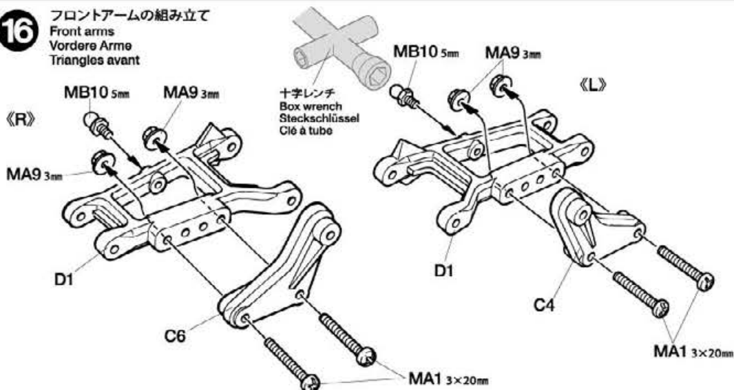
MB10 ×2 5mmビローボール Ball connector Kugelpopf Connecteur à rotule
