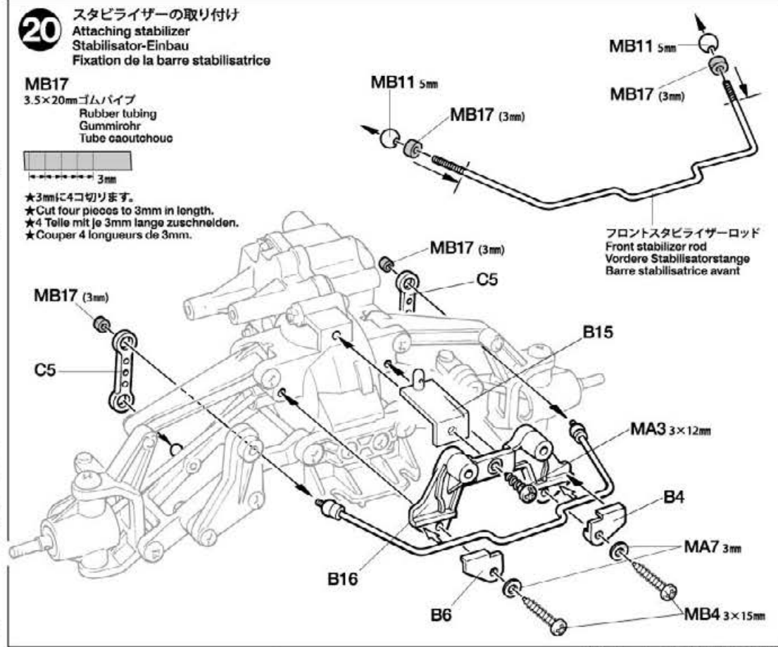
MB4 x2 3×15mm タッピングビス Tapping screw Schneidschraube Vis taraudeuse
