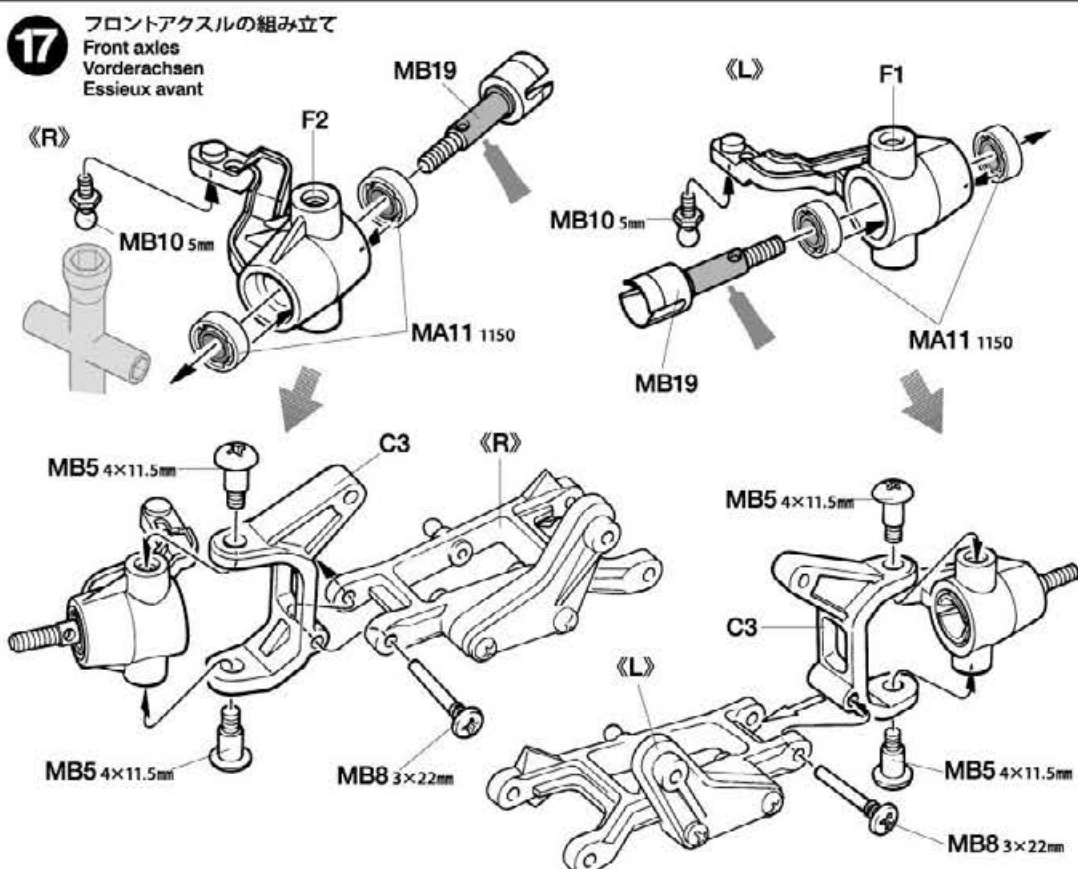
MB10 ×2 5mmビローボール Ball connector Kugelpopf Connecteur à rotule
