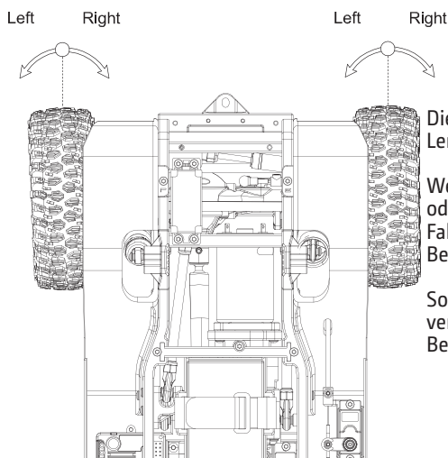
Lenkungsstrimmung
