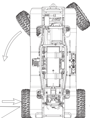
In diesem Modus wird beim nach links Lenken das linke hintere Rad abgebremst.
