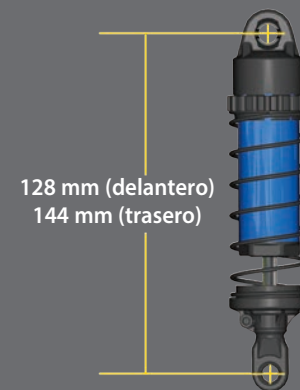
Tama±os de pist3n de amortiguador
