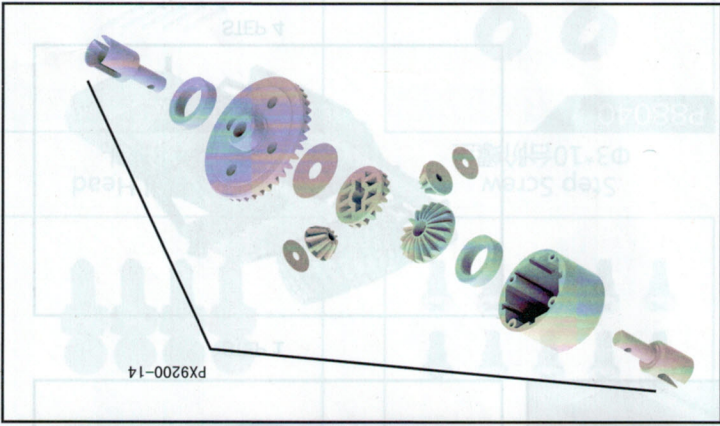
合金差速器组装图
