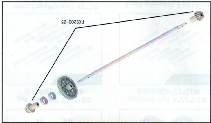
传动轴总成分解图
