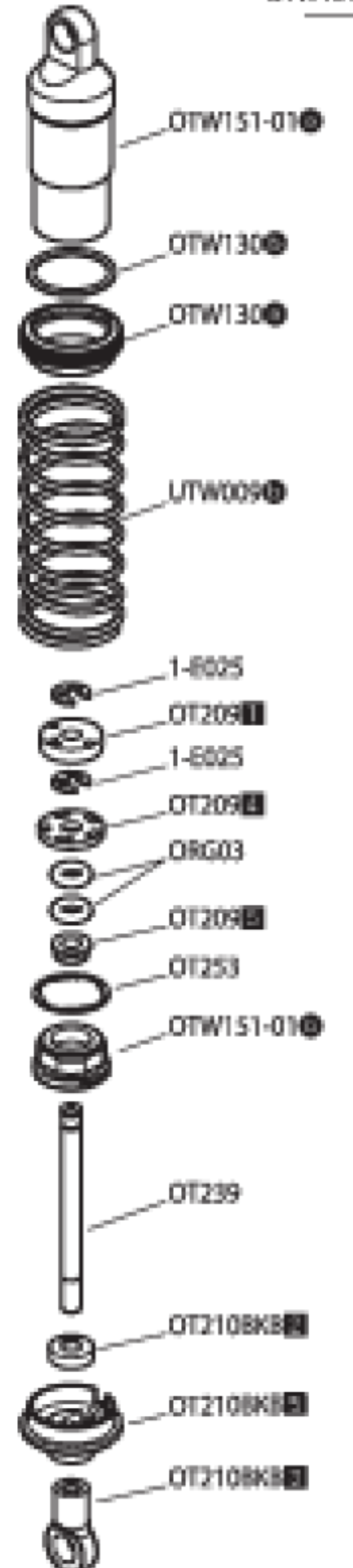
Front Shock フロントショック OTW151
