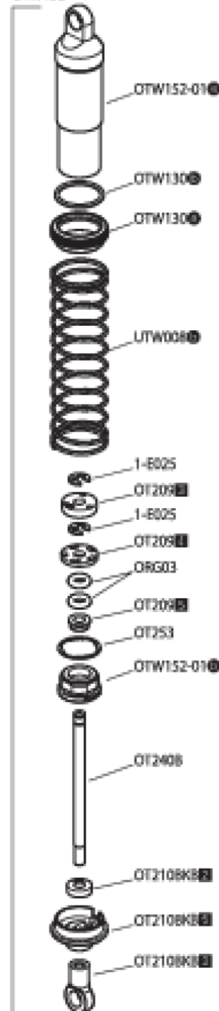
Rear Shock リヤショック OTW152
