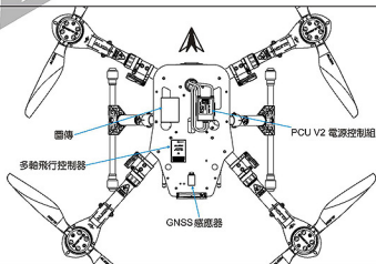
電子設備配置示意圖
