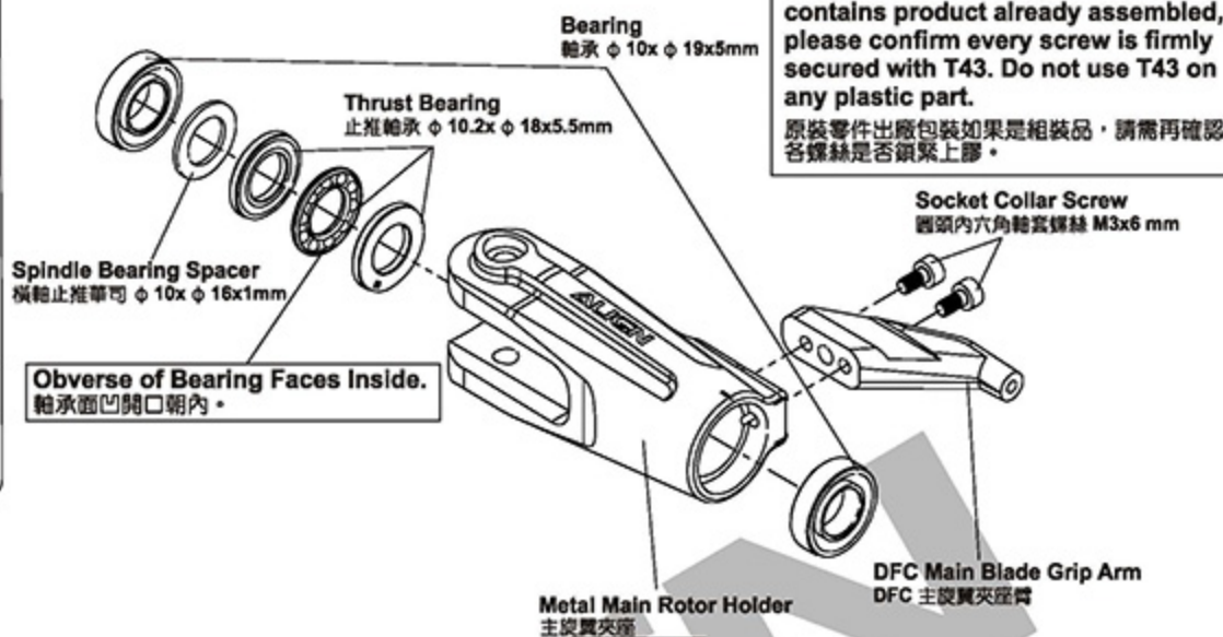
Spindle Bearing Spacer 橫軸止推華司 (φ 10x φ 16x1mm) x 2
