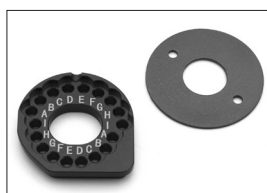
FAW217 ★1870 HD モーターマウント (FZ02全車種) HD Motor Mount (FZ02)
