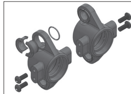
FAW205 HDフロントハブ FZ02 (2個入) HD Front Hub FZ02 (2pcs)
